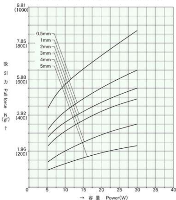
標準コイル表 定格 5.3W Standard Coil Specifications Rated Power 5.3W
