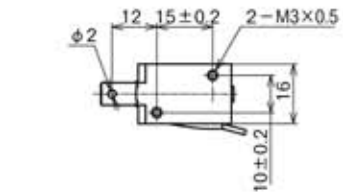
外形寸法 Dimensions
